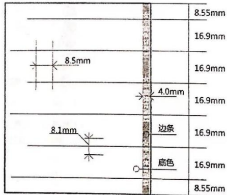
图 A.2 热敏涂层版面图案 B
