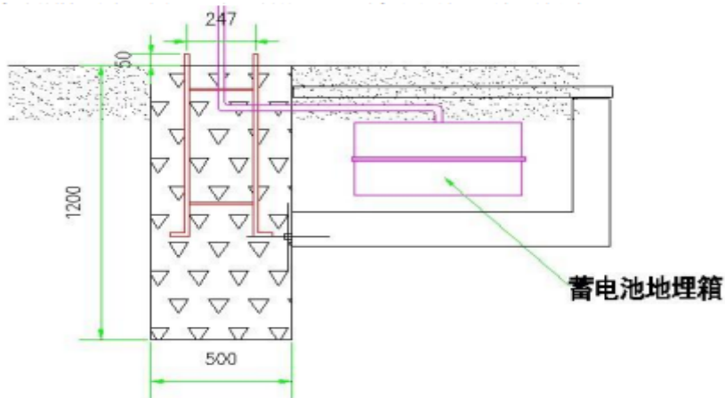
6米太阳能监控杆基础剖面图
