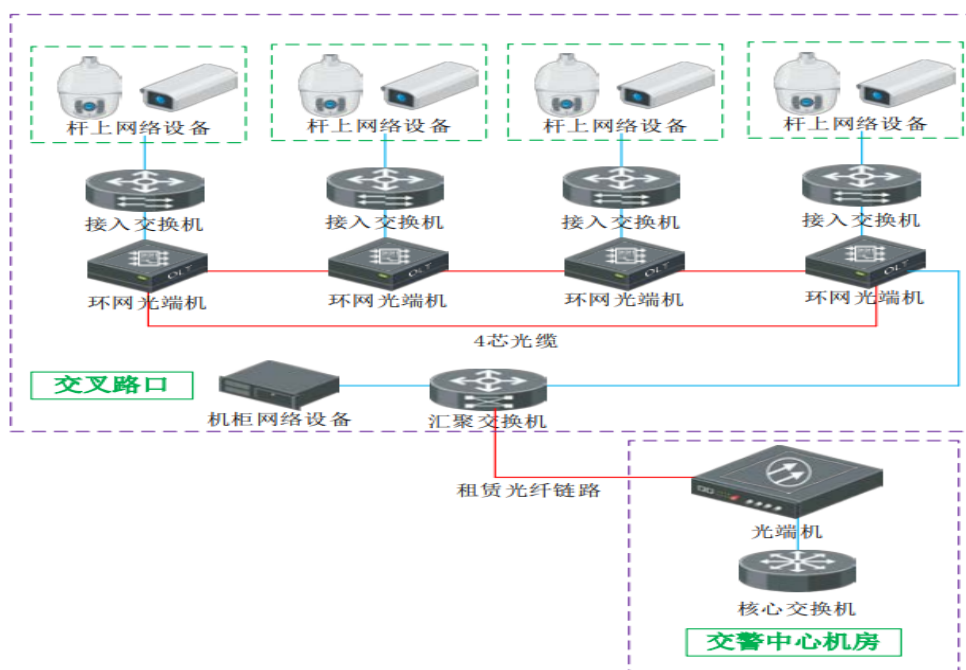
网络传输系统图
